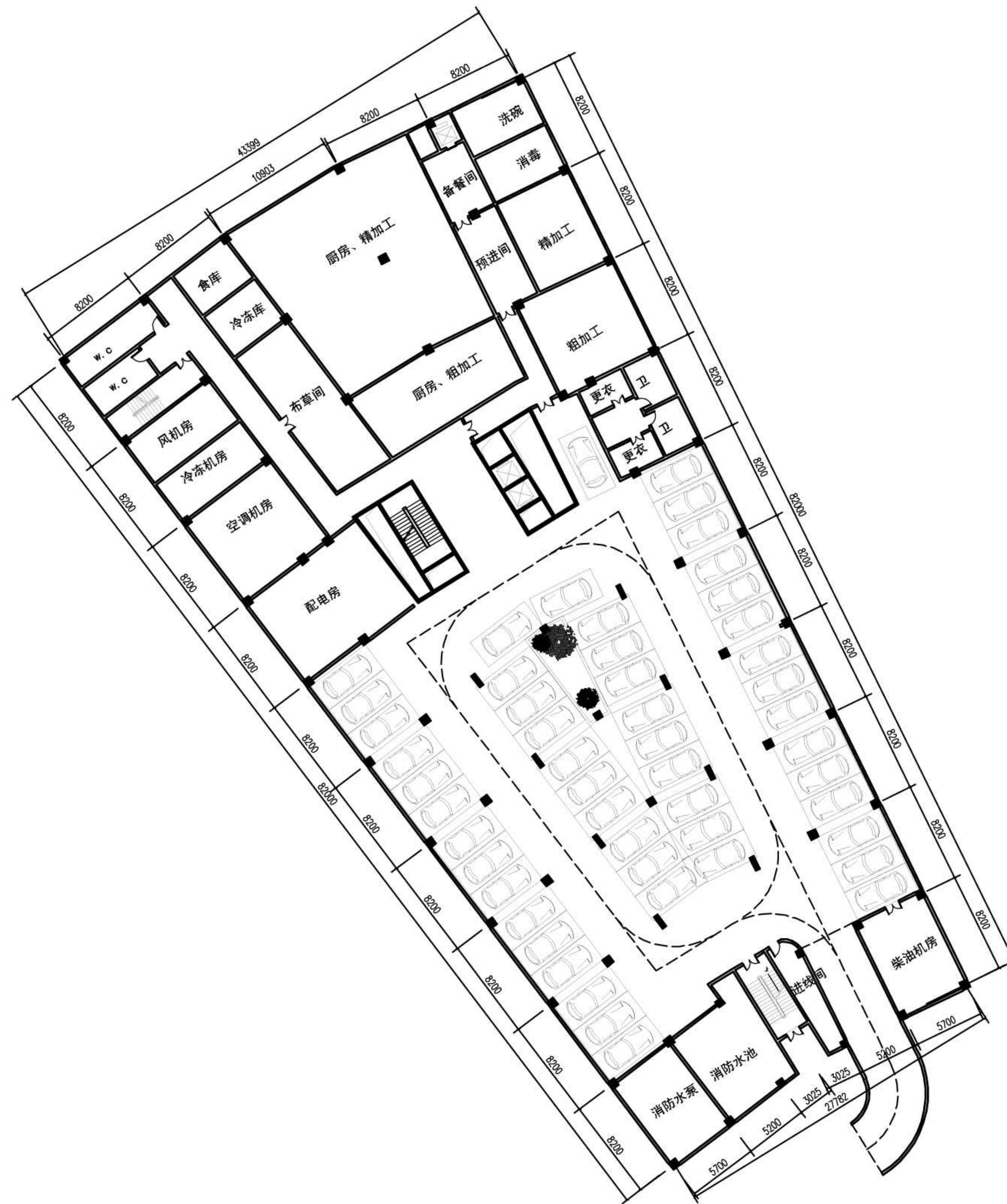
level -1f 负一层平面图 1:300 (地下车库车位: 48)
