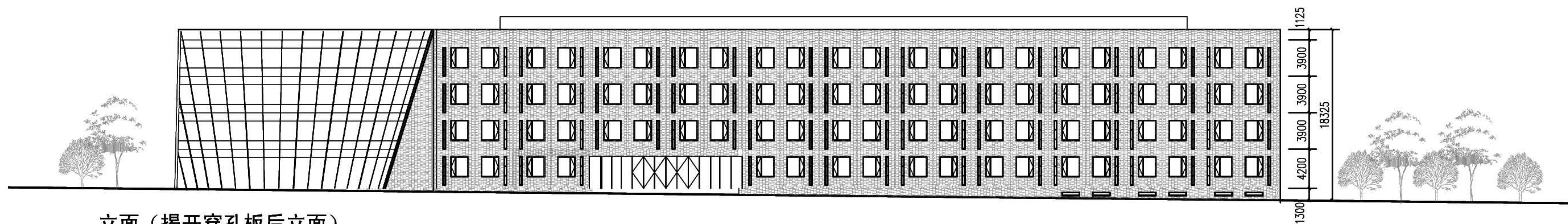
立面 (揭开穿孔板后立面)
